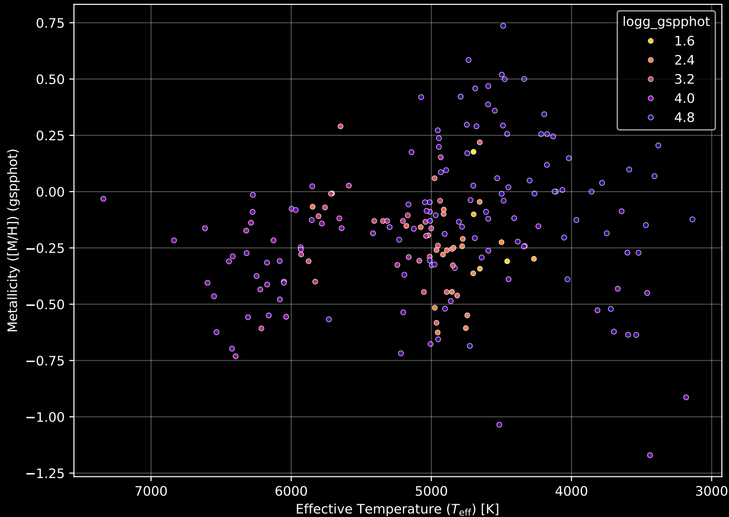
APOGEE DR17 Field: [200+60] Stellar Population Parameters (n= 195)
